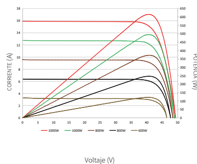
Curvas de corriente-voltaje y potencia-voltaje (615W)
